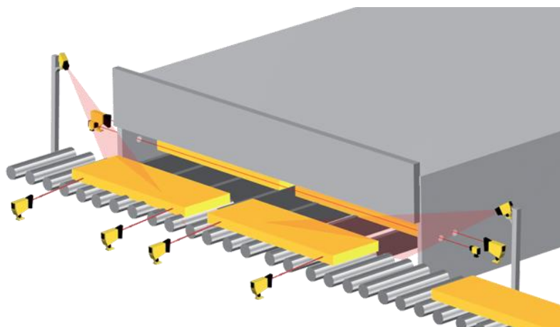
加热炉出炉侧的双排料板坯的检测与位置控制
